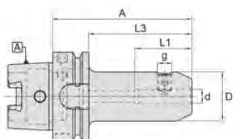
Aufnahme HSK-A63 für Schafffräser / Weldon Chuck HSK-A63 for end milling cutter / Weldon
