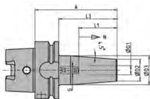
Aufnahme HSK-A63 für Schafffräser / Schrumpffutter Chuck HSK-A63 for end milling cutter / Shrink Chucks
